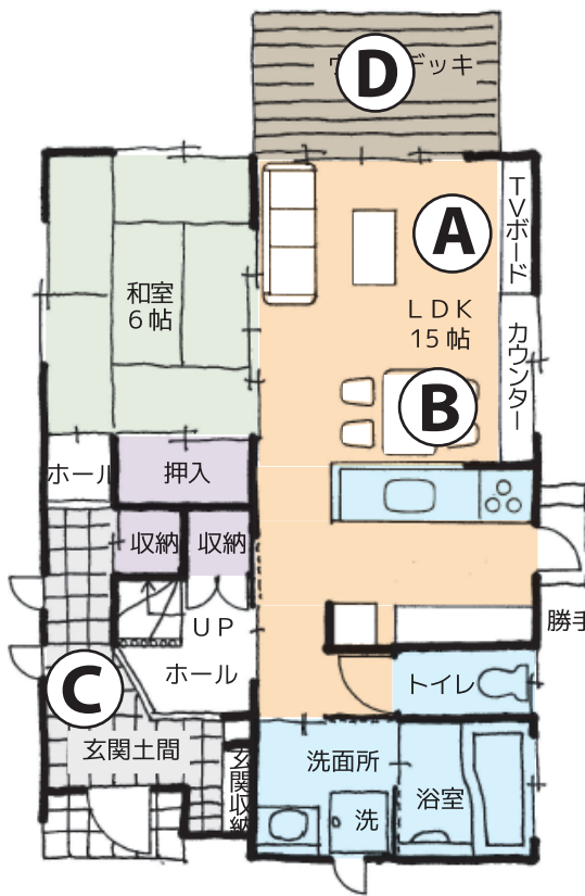
1階平面図
